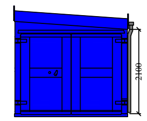
END ELEVATION
