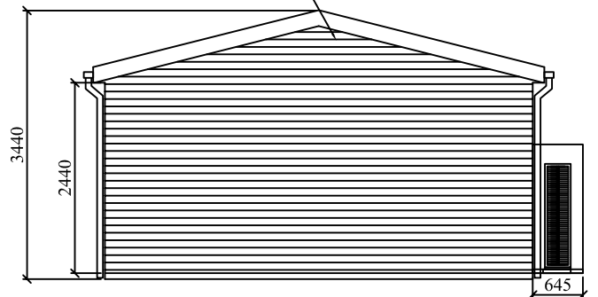
END ELEVATION
